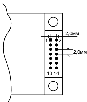
Рис. 1. Разводка выходного НЧ соединителя
